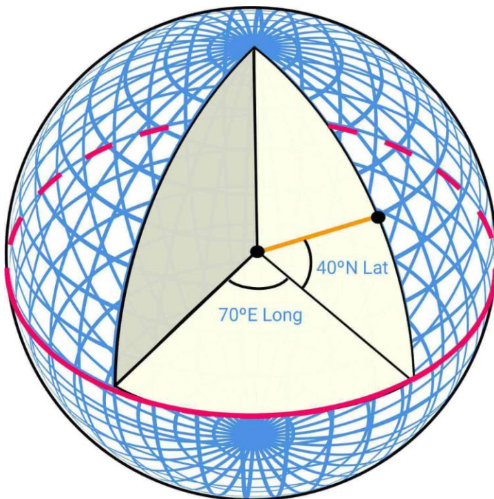
Figure 1 Latitude and Longitude (source: [5])
